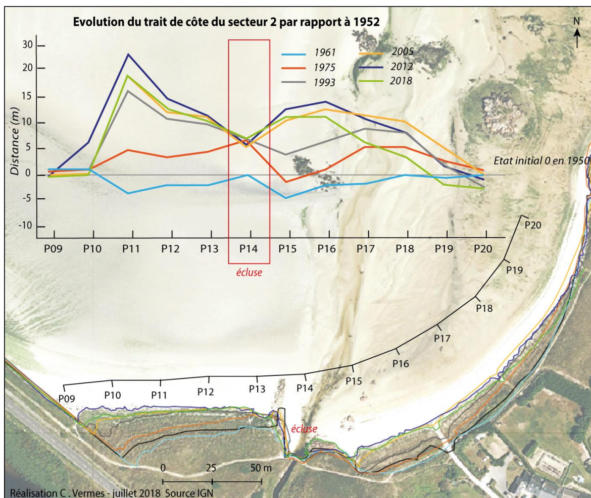
Figure 18. Analyse de la cinématique du trait de côte du secteur 2
