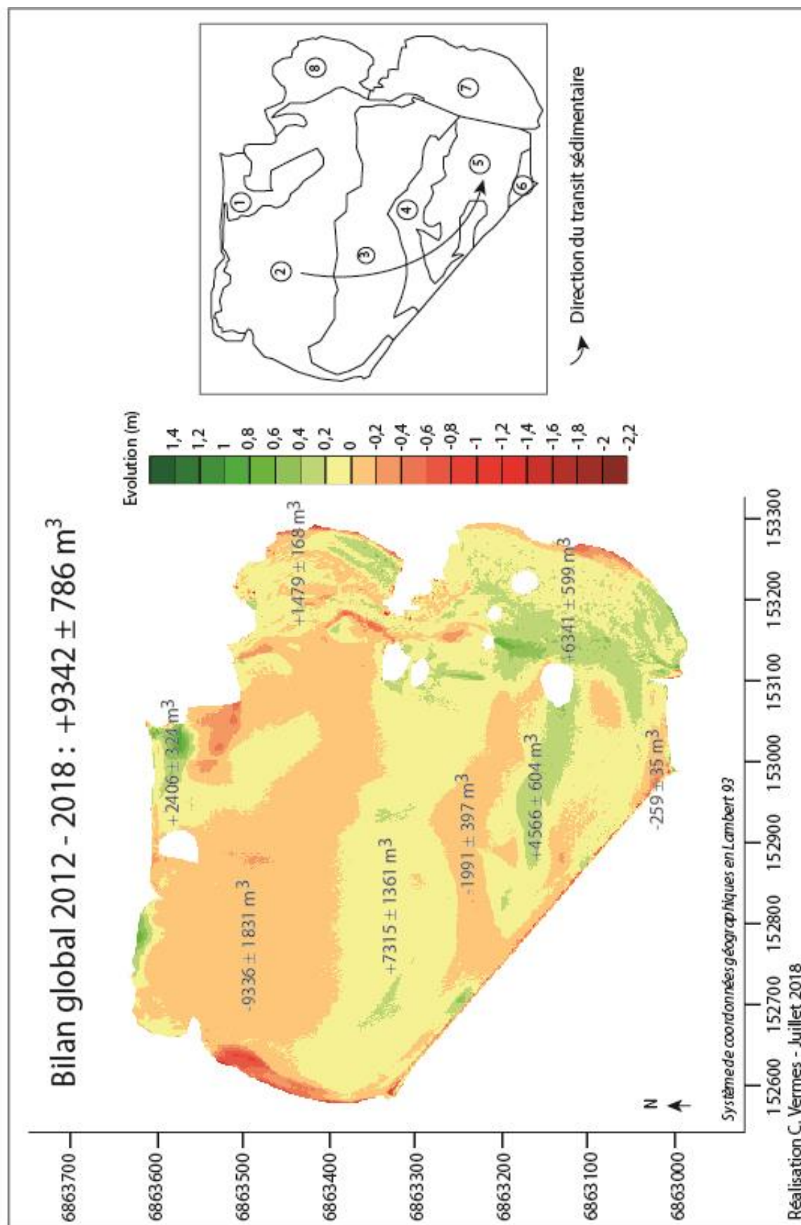
Figure 21. Modélisation du bilan sédimentaire de la baie de Porz Olier entre 2012 et 2018
